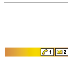
Рис. 3 Экранная заставка
